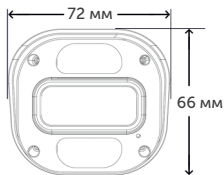
Рис.1 Вид спереди
