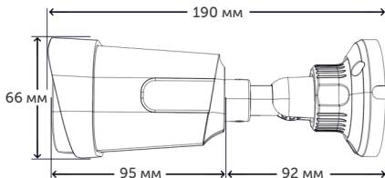
Рис.2 Вид сбоку
