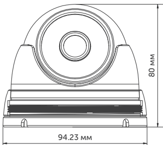
Рис.2 Вид сбоку
