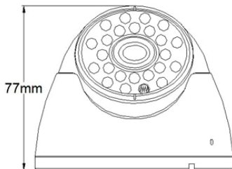
Рис.2 Вид сбоку
