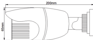
Рис.1 Вид сбоку
