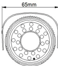
Рис.2 Вид сверху
