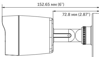
Рис.2 Вид сбоку
