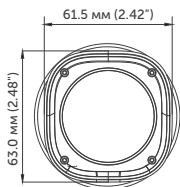
Рис.1 Вид спереди
