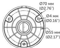
Рис.3 Крепление
