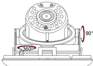
Рис.1 Вид спереди
