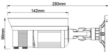
Рис.1 Вид сбоку
